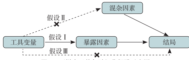
图1 两样本孟德尔随机化假设示意图
