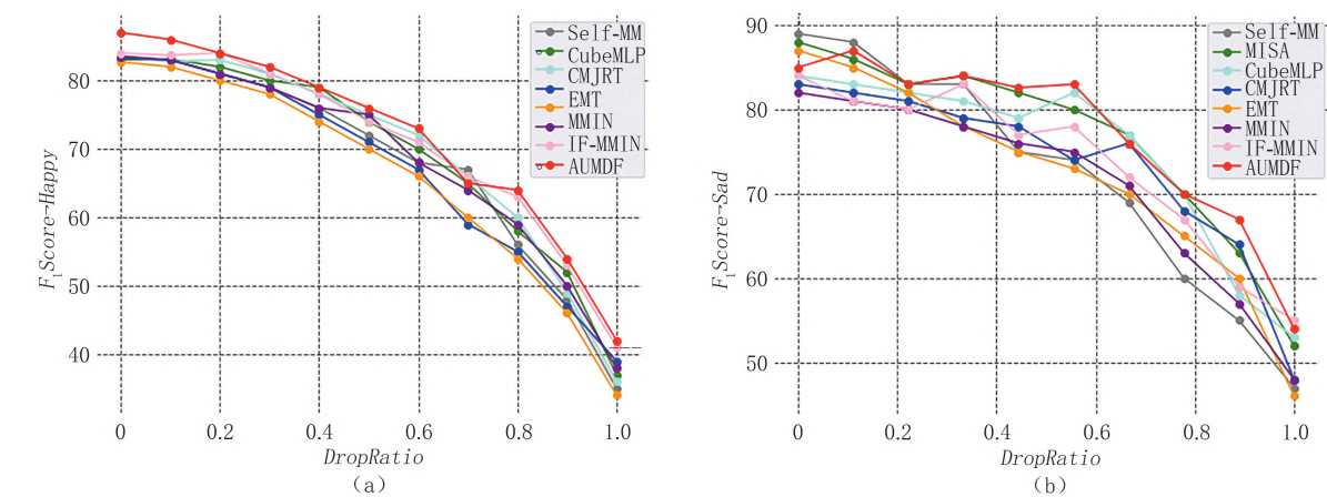
图5 不同丢失率设置下在IEMOCAP数据集上的实验结果
