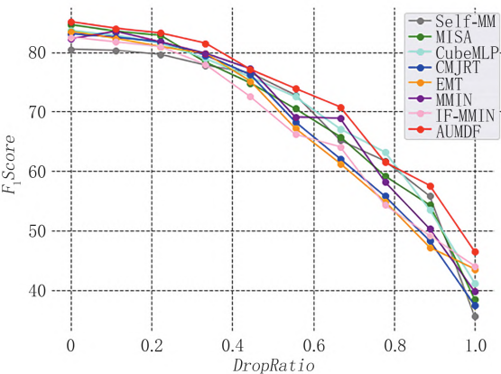
图6 不同丢失率设置下在CMU-MOSEI数据集上的实验结果
