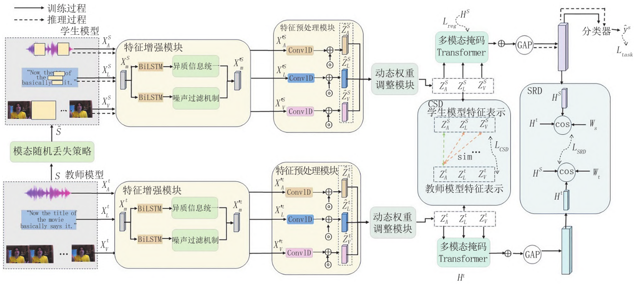
图1 AUMDF 结构框架
