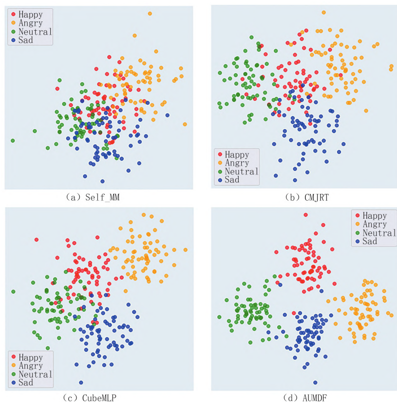
图7 在IEMOCAP测试集上的可视化结果
