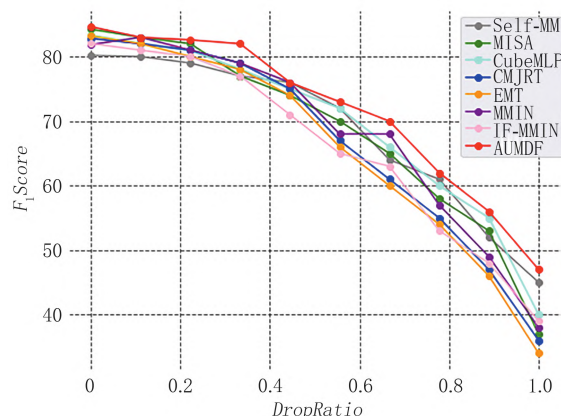
图4 不同丢失率设置下在CMU-MOSI数据集上的实验结果
