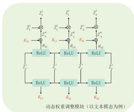
图2 动态权重调整模块架构
