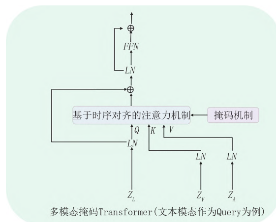
图3 多模态掩码 Transformer 架构
