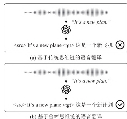
图 1 基于鲁棒思维链的语音翻译示意图
